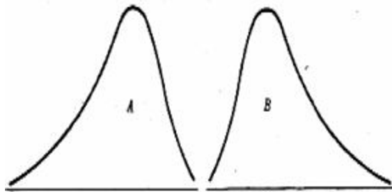
Fig. 6. Curvas oblicuas
